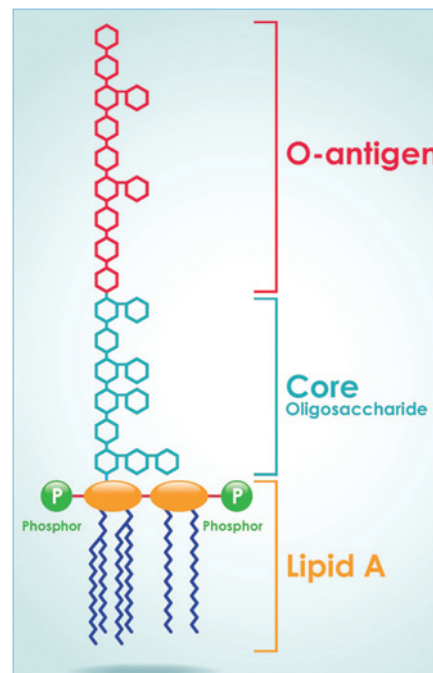
Fig. 1. LPS molecule.
